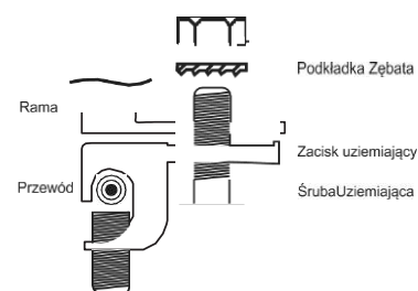
Rys. 7: Metody instalacji
